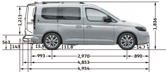
Caddy Maxi 尺寸圖
